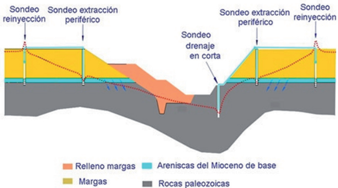
Figura 3.15 Modelo de Bombeo – Reinyección en Cobre las Cruces. (CLC, 2008)
