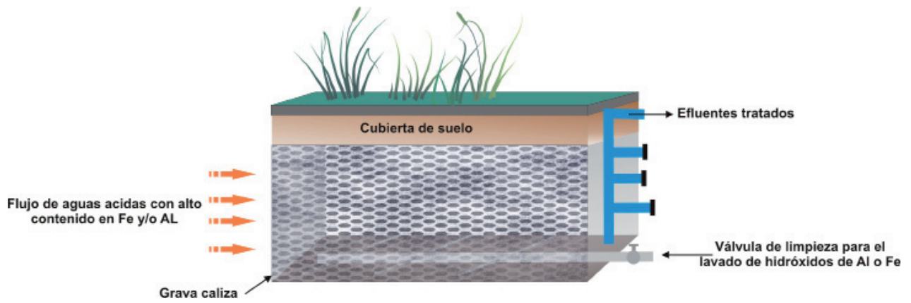
Figura 5.6 Esquema de un OLC
