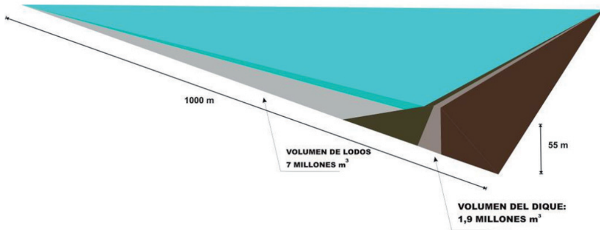
Figura 3.35 Esquema de una sección de una balsa convencional.
