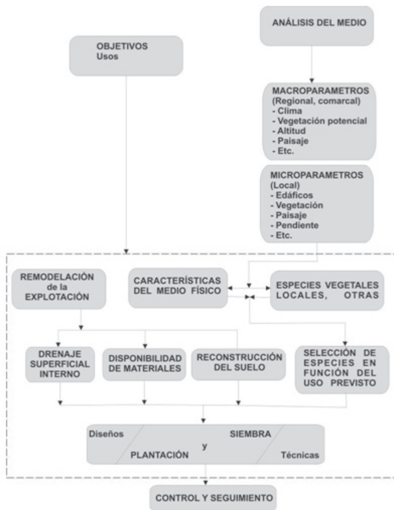
Figura 3.44 Factores del Medio Físico a Tener en Cuenta y Acondicionamiento del Terreno para Instaurar un uso Determinado. (Ayala, 2004)
