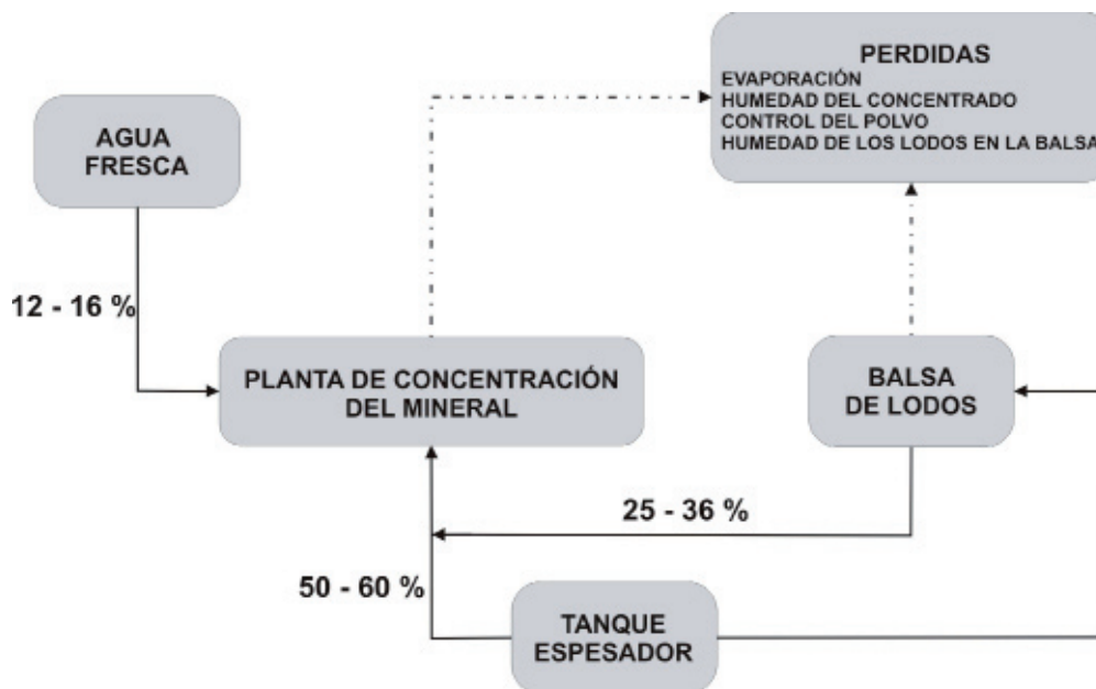
Figura 3.12 Ejemplo de un Balance de Agua por Componente
