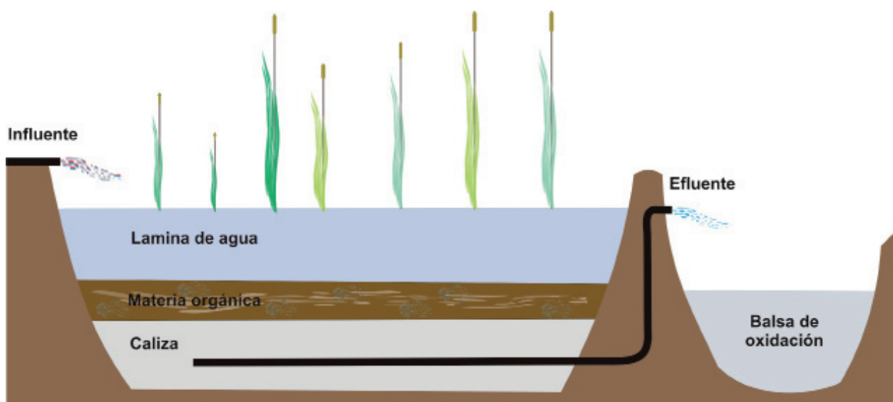
Figura 5.8 Esquema del Sistema RAPS
