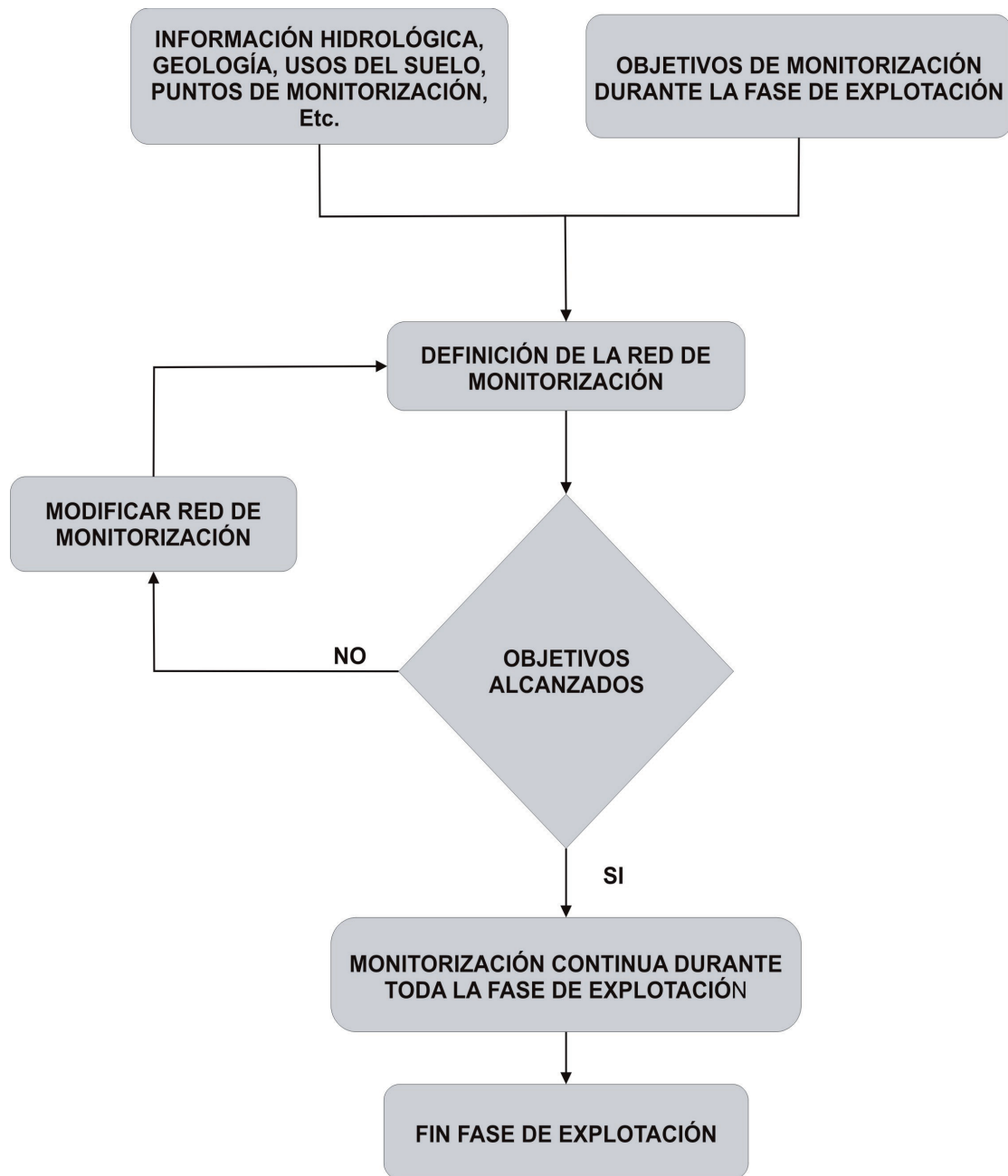
Figura 2.7 Esquema de la Fase de Monitorización durante la Explotación de la Mina
