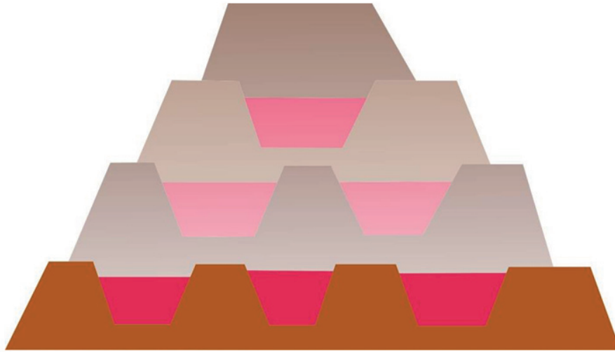
Figura 3.21 Esquema de una Escombrera con Disposición Selectiva de los Materiales.
