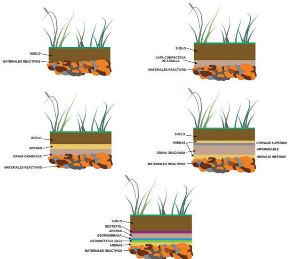
Figura 3.40 Distintos Tipos de Coberturas Secas
