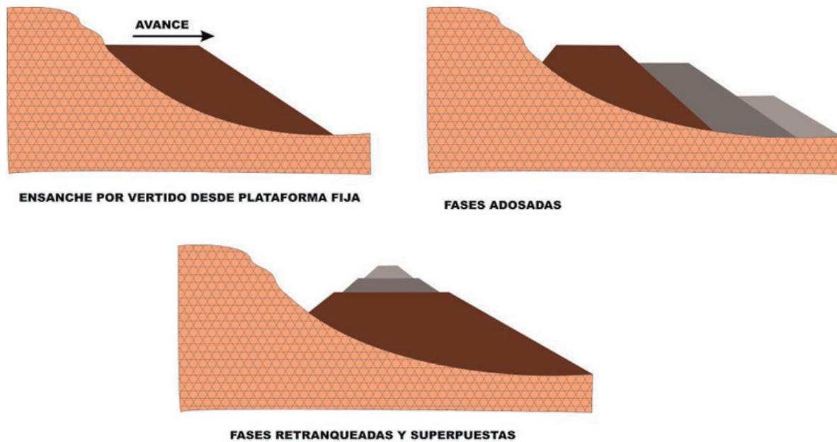
Figura 3.19 Formación de Escombreras
