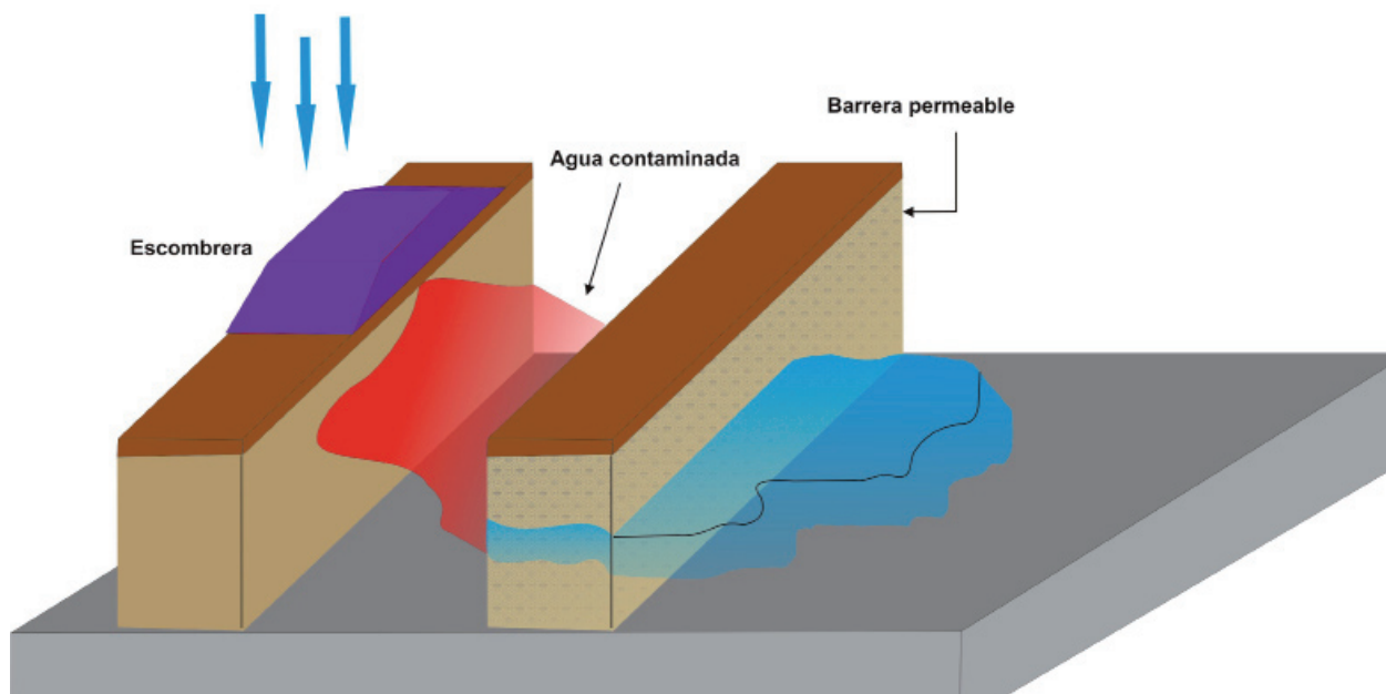
Figura 5.7 Esquema de una Barrera Permeable
