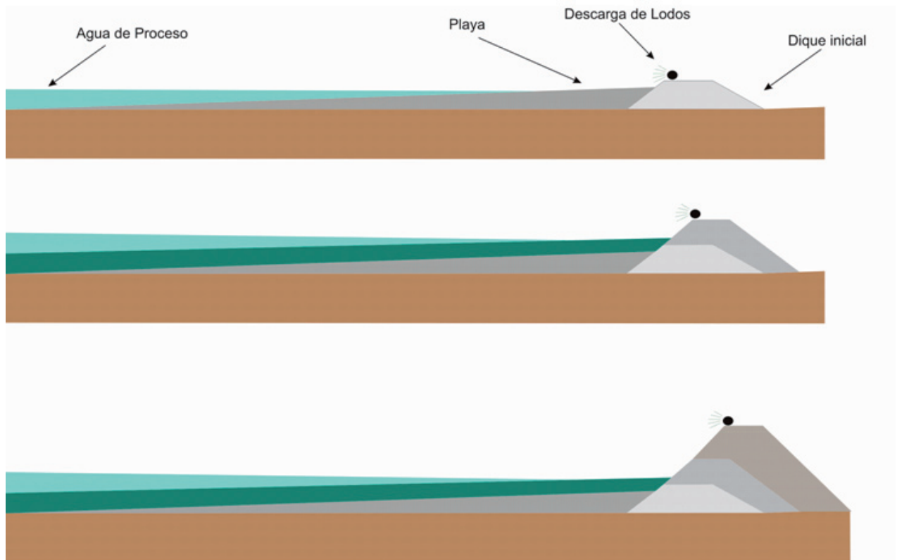
Figura 3.27 Esquema de Construcción de una Balsa por el Método de Línea Central
