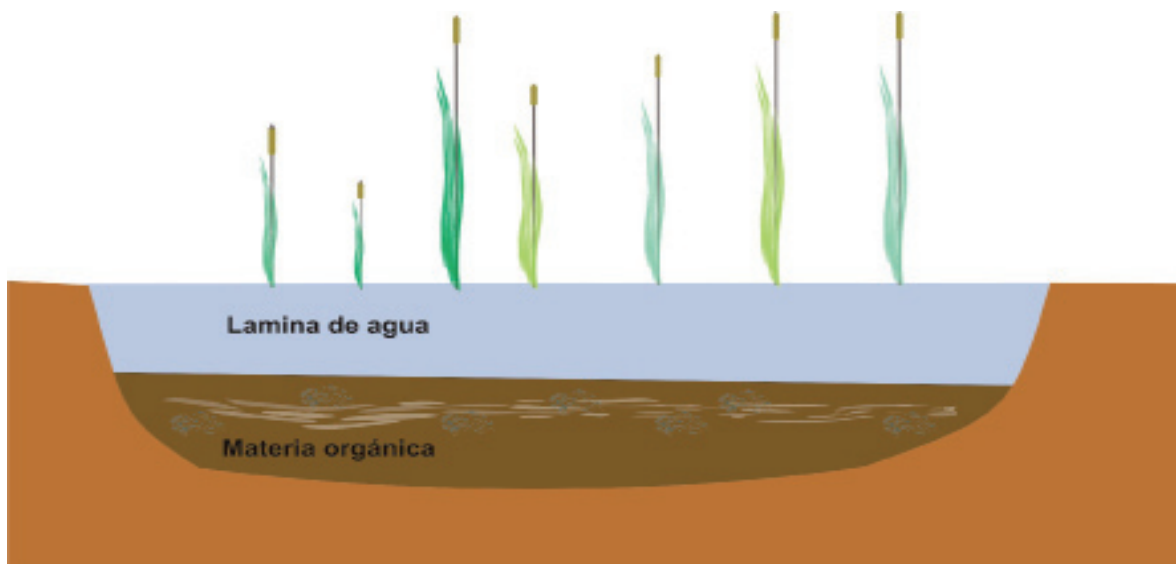
Figura 5.3 Esquema de un Humedal Anaerobio o de Sustrato Orgánico
