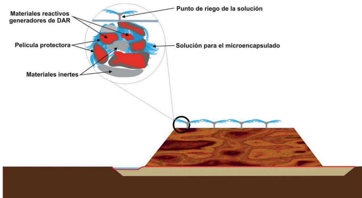
Figura 3.23 Esquema del Proceso de Microencapsulado de Materiales Reactivos.
