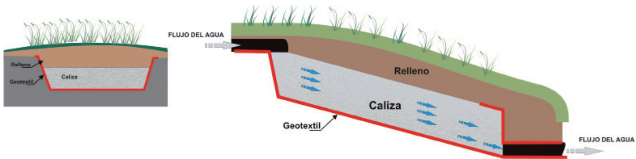
Figura 5.4 Esquema de un ALD
