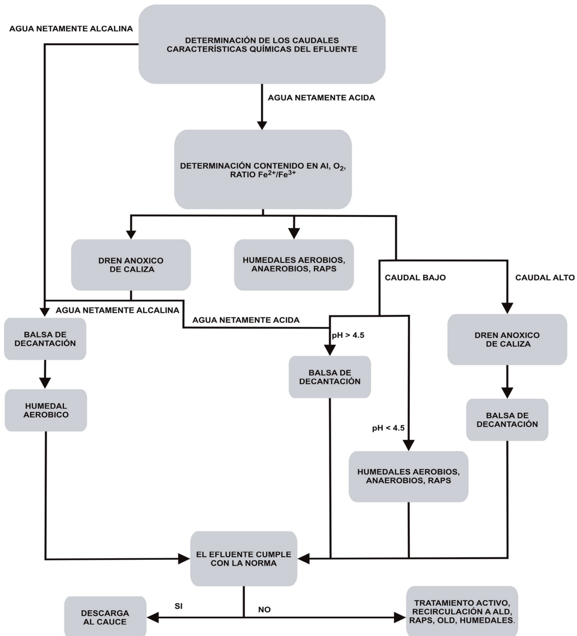
Figura 5.1 Esquema del diagrama de flujo para la Selección de Tratamientos Pasivos de Aguas Ácidas. Basado en Younger et al, 2002 y Wolkersdorfer, 2006
