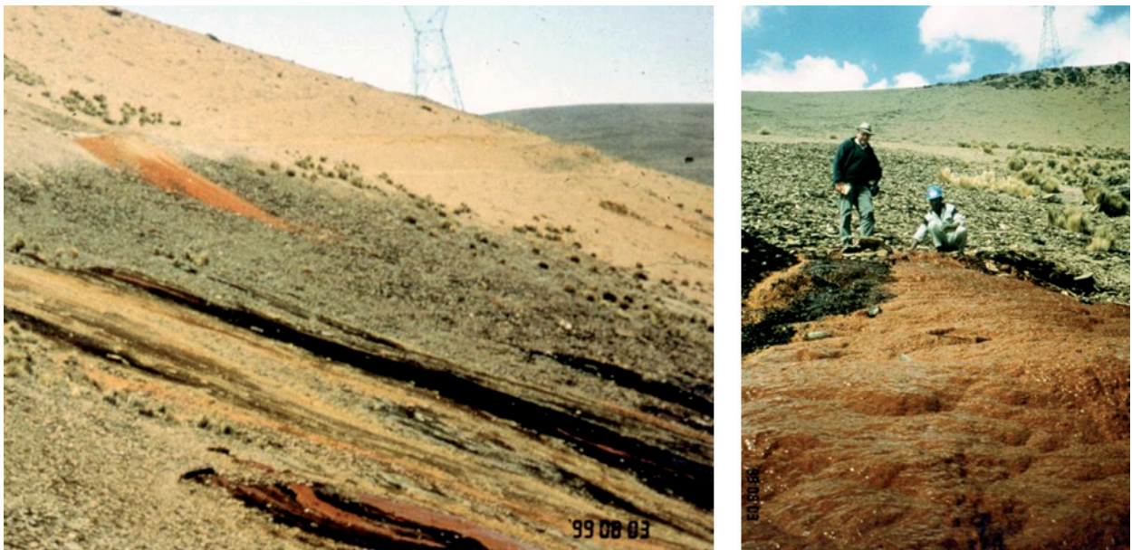
Figura 3.8 Sondeos de Exploración Abandonados sin Sellar, descargando Aguas Ácidas de Mina (Fotos: P. L. Younger)
