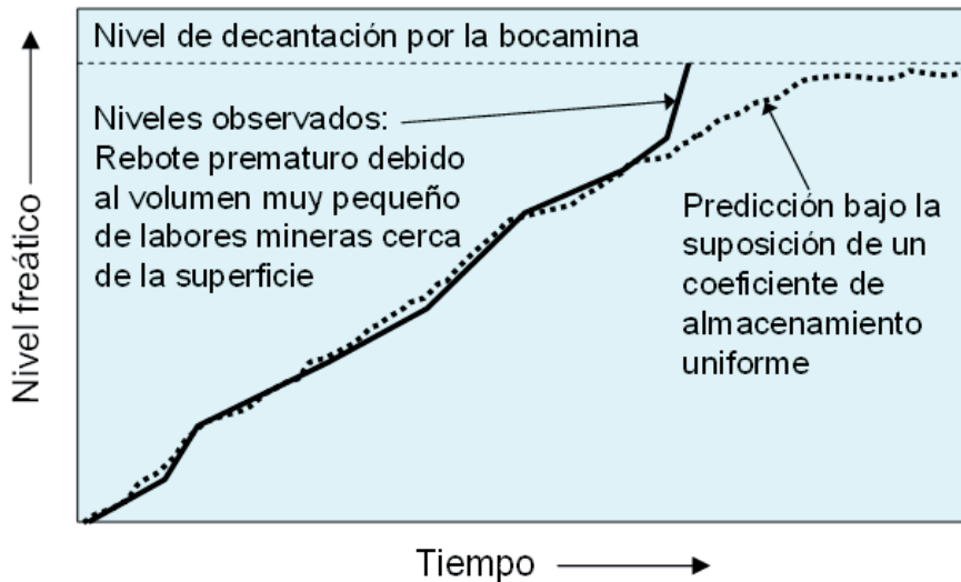
Figura 3.42 Rebote de Agua en una Mina Subterránea tras el Cierre
