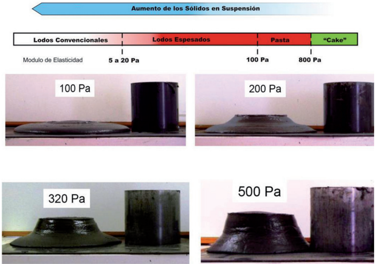
Figura 3.37 Tipos de Lodos en Función de su Contenido en Sólidos. Modificado de Cooke, 2008.
