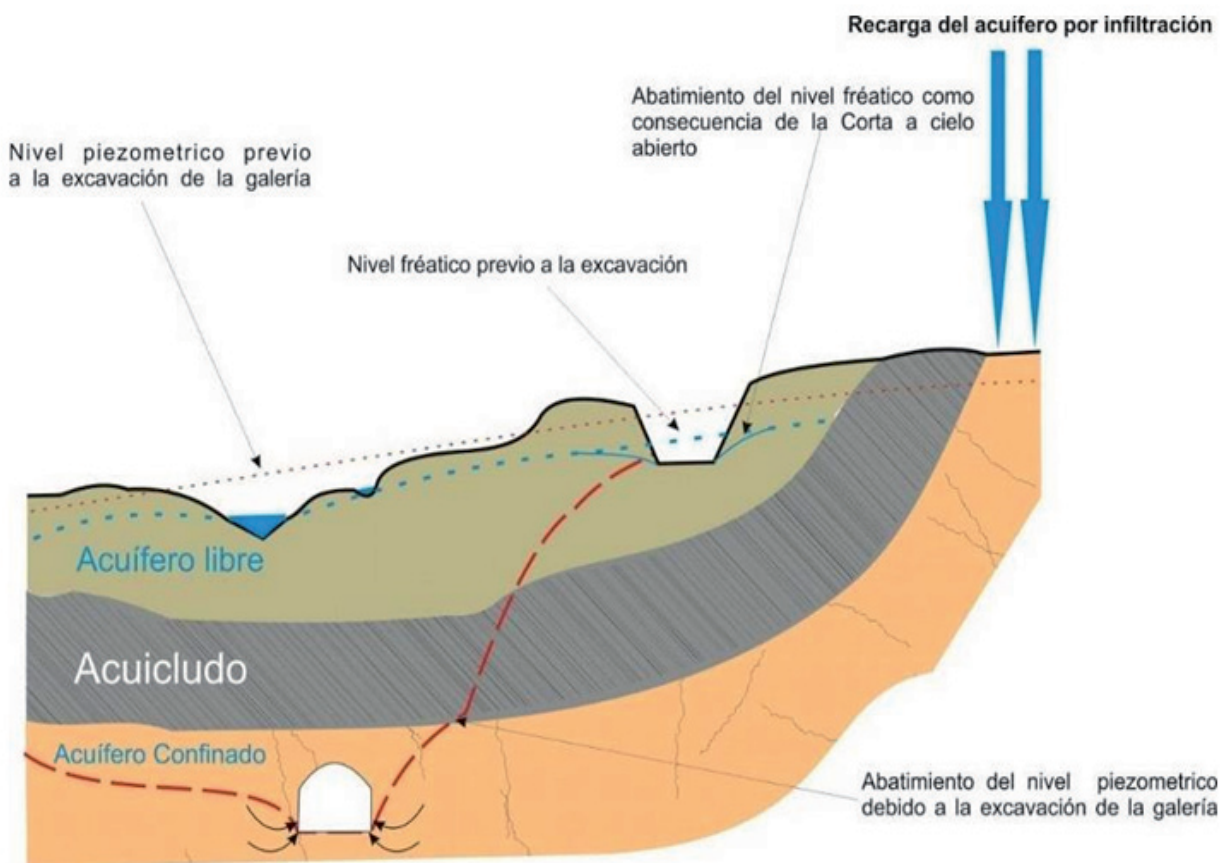
Figura 3.7 Modificación de los niveles freáticos y piezométricos debidos a la actividad minera
