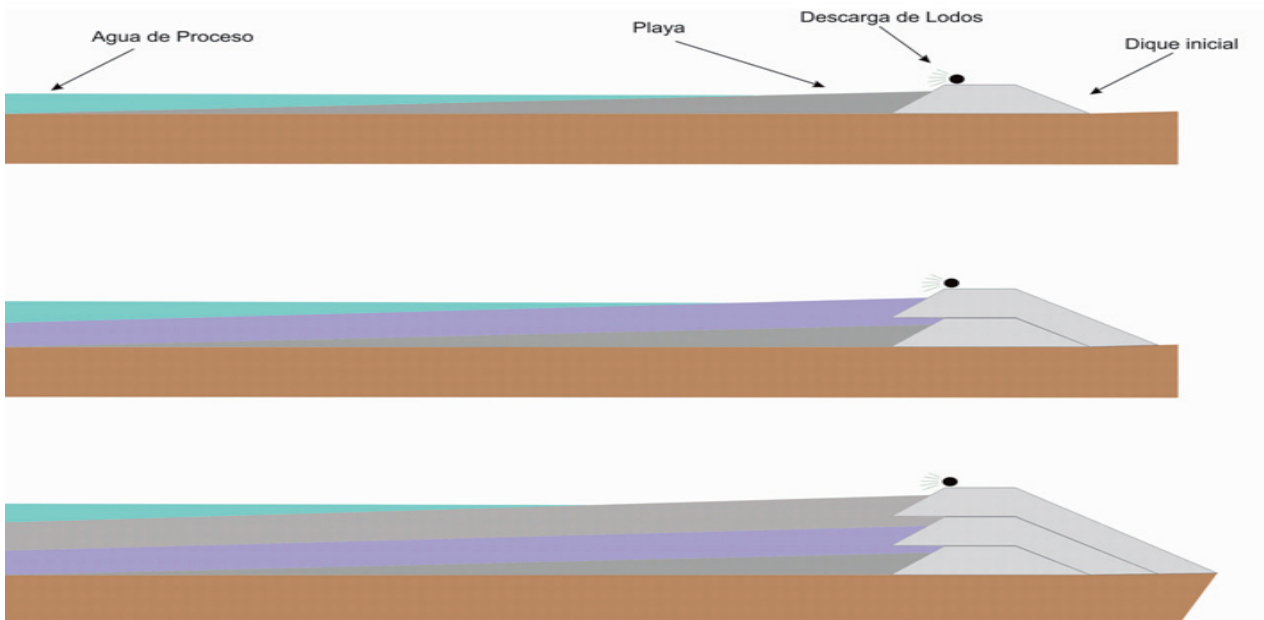
Figura 3.26 Esquema de Construcción de una Balsa por el Método Aguas Abajo
