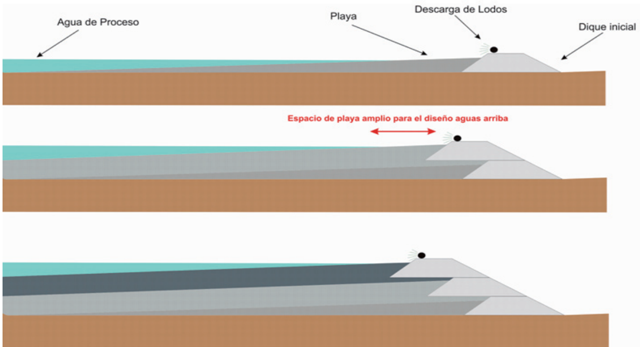
Figura 3.25 Esquema de Construcción de una Balsa por el Método Aguas Arriba (nota: método prohibido en Chile, Perú y otros países por su inestabilidad inherente durante eventos sísmicos)
