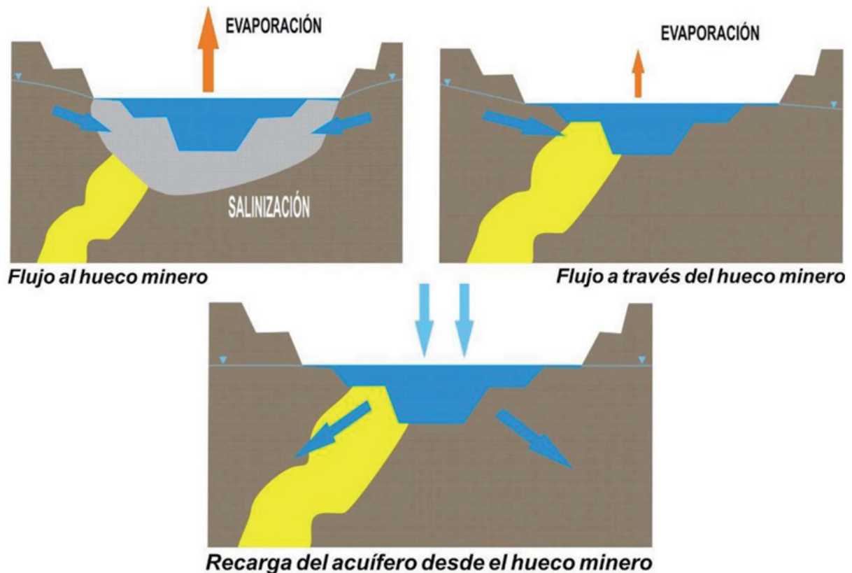
Figura 3.9 Tipología de Huecos Mineros Inundados. (Basado en Fernández, 1998; Younger et al., 2002)
