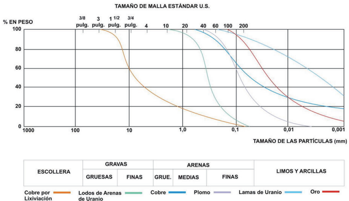
Figura 3.24 Curvas Granulométricas Tipo para Diferentes Metales Tratados (Ayala, 2004)
