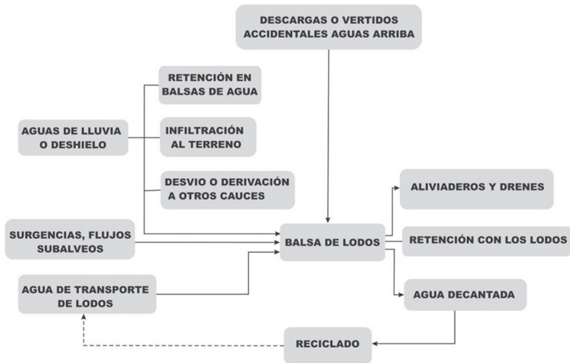
Figura 3.29 Procedencia y Flujo del Agua en las Balsas de Lodos
