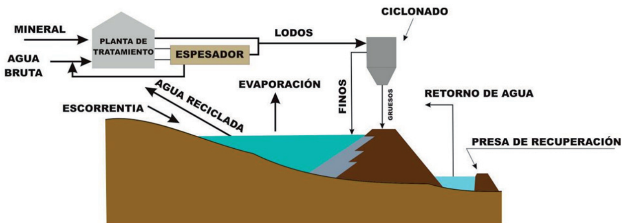
Figura 3.32 Ciclo del Agua en una Planta de Tratamiento de Minerales (modificado de Ayala, 2004).
