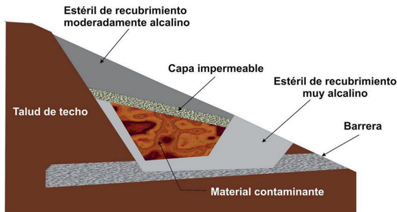
Figura 3.20 Vertido Selectivo de los Materiales. Basado en Ayala, 1996
