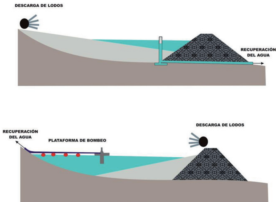
Figura 3.33 Modos de Recuperación del Agua de las Balsas de Lodos. Punto central (arriba), Plataforma móvil (abajo). (modificado de Ayala, 2004)
